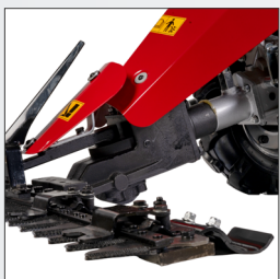
Falciatrice manovellismo in bagno d'olio
